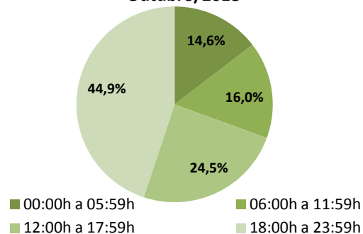
Gráfico 03: Percentual de CVLI por turno - Outubro/2018
