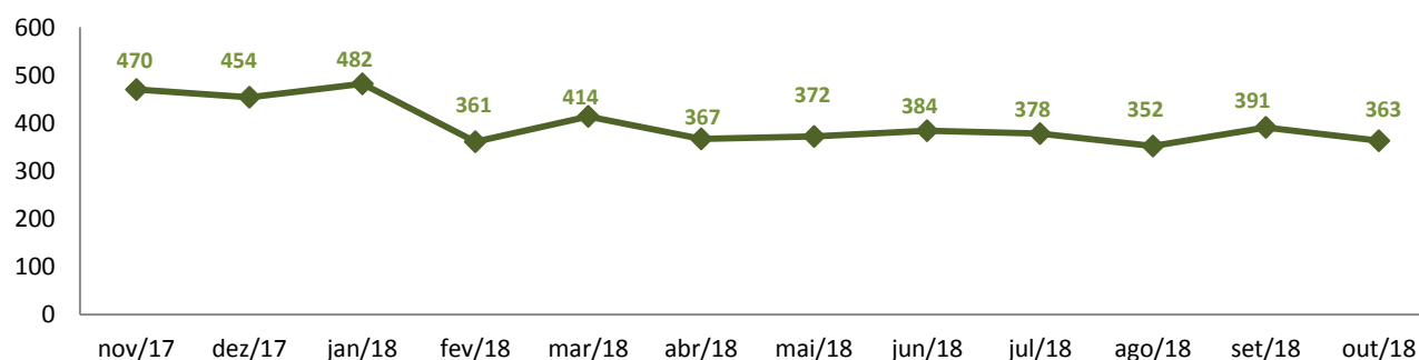
Gráfico 01: Série mensal de CVLI no Ceará
