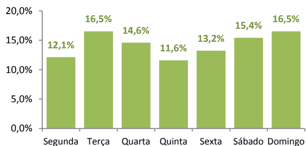
Gráfico 02: Percentual de CVLI por dia da semana - Outubro/2018
